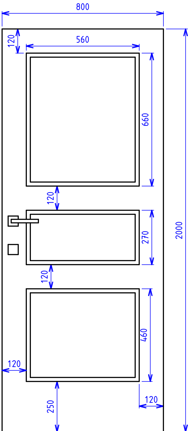
PORTA STANDARD - TIPO 1
