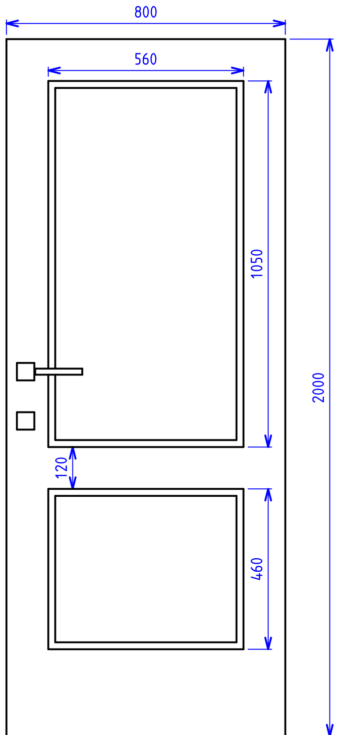
PORTA STANDARD - TIPO 2
